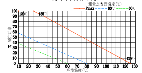
功率降额曲线
